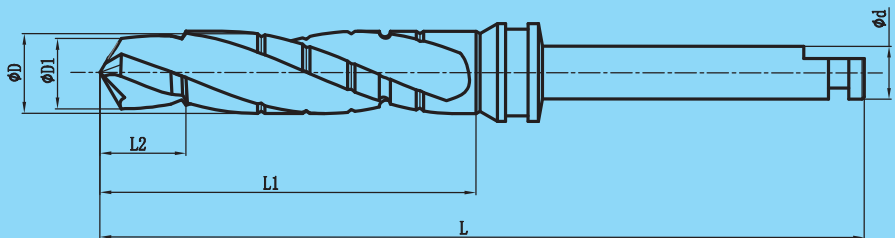
部分尺寸 some size
