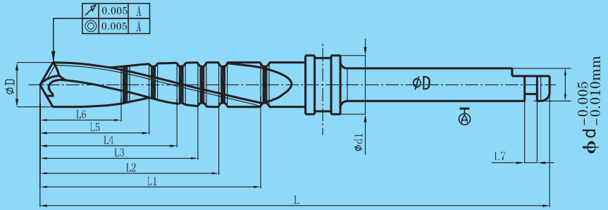
部分尺寸 some sizes
